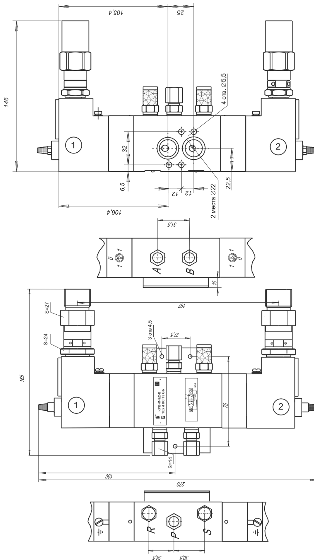
Рисунок 2.4 - Габаритные и установочные размеры пятиходовых бистабильных исполнений клапана КРВ-М-5/2-6-В**
