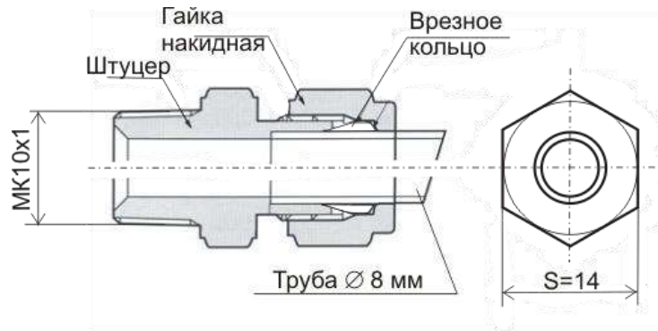
Рисунок 7.5 - Конструкция соединения А-8-MLL
